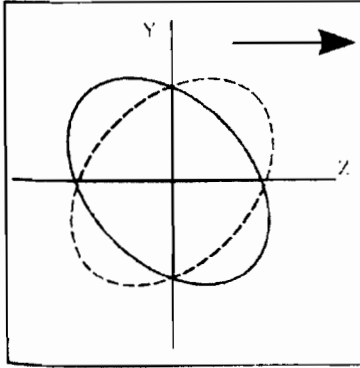
E- الحالة الأولى لاستقطاب الموجة التجاذبية الصريف
